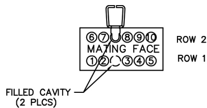
PLUG MA-231-010-161-ABCWA
