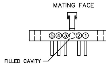
RECEPTACLE MA-181-005-435-A0300
