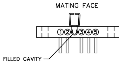
PLUG MA-171-005-325-A0300
