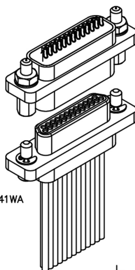
MMHT-223-025-2A3-2200 (METAL)
