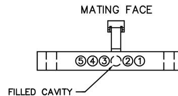
RECEPTACLE MA-121-005-261-A03WA
