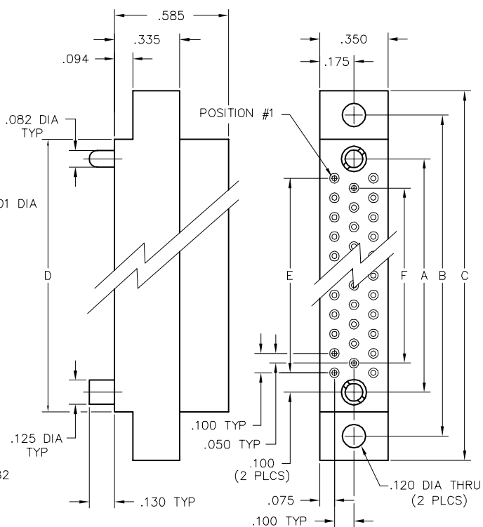
RECEPTACLE
