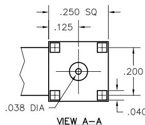
VIEW A-A
